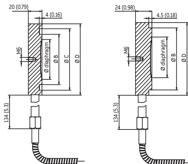
EN 1092-1 Form D
