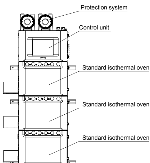
Type 3 (Wall-mounting)
